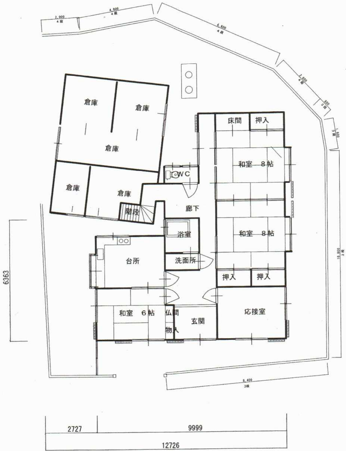
1階現況平面図
